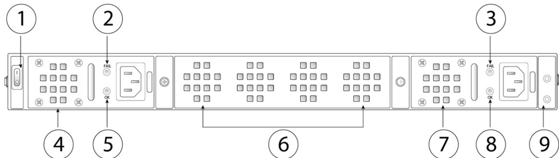
Figura 10: Panel trasero de Firepower 2130 y 2140
