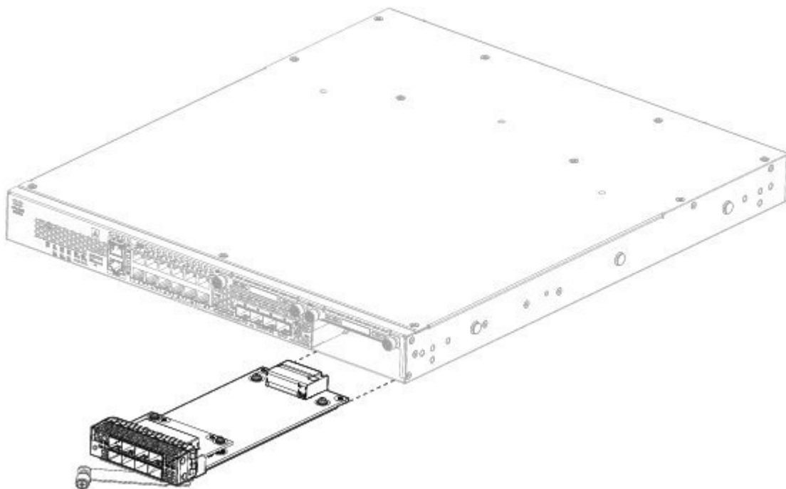
Figura 20: Extracción del módulo de red de Firepower 2130 y 2140
